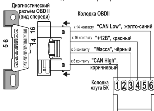
Рис.2 Схема подключения БК "ШТАТ Х1-С"
